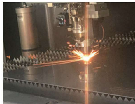
加工の様子
