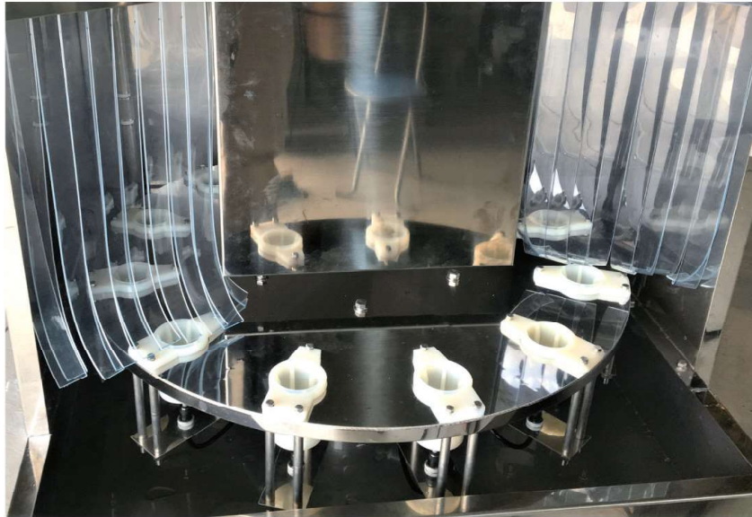
洗びん装置
