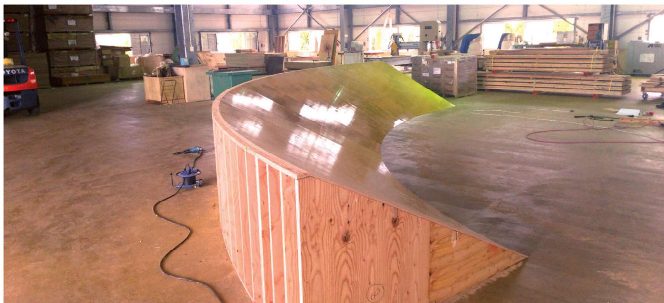
円錐型枠
