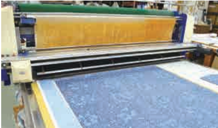
延反機
