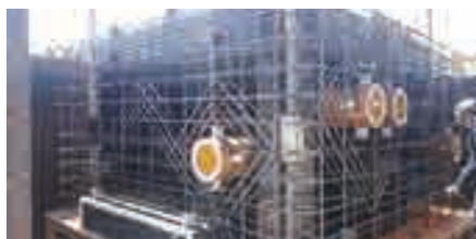
ボックスカルバート製造状況
