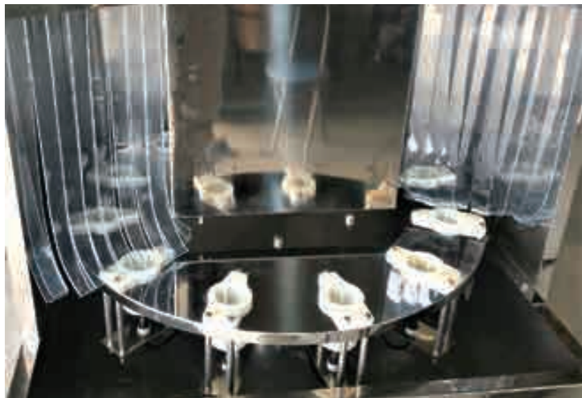
洗びん装置
